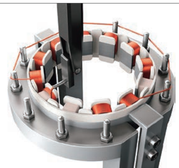
モータ 巻線工程
