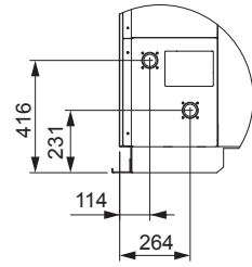
冷水回路部詳細(公差±5)
