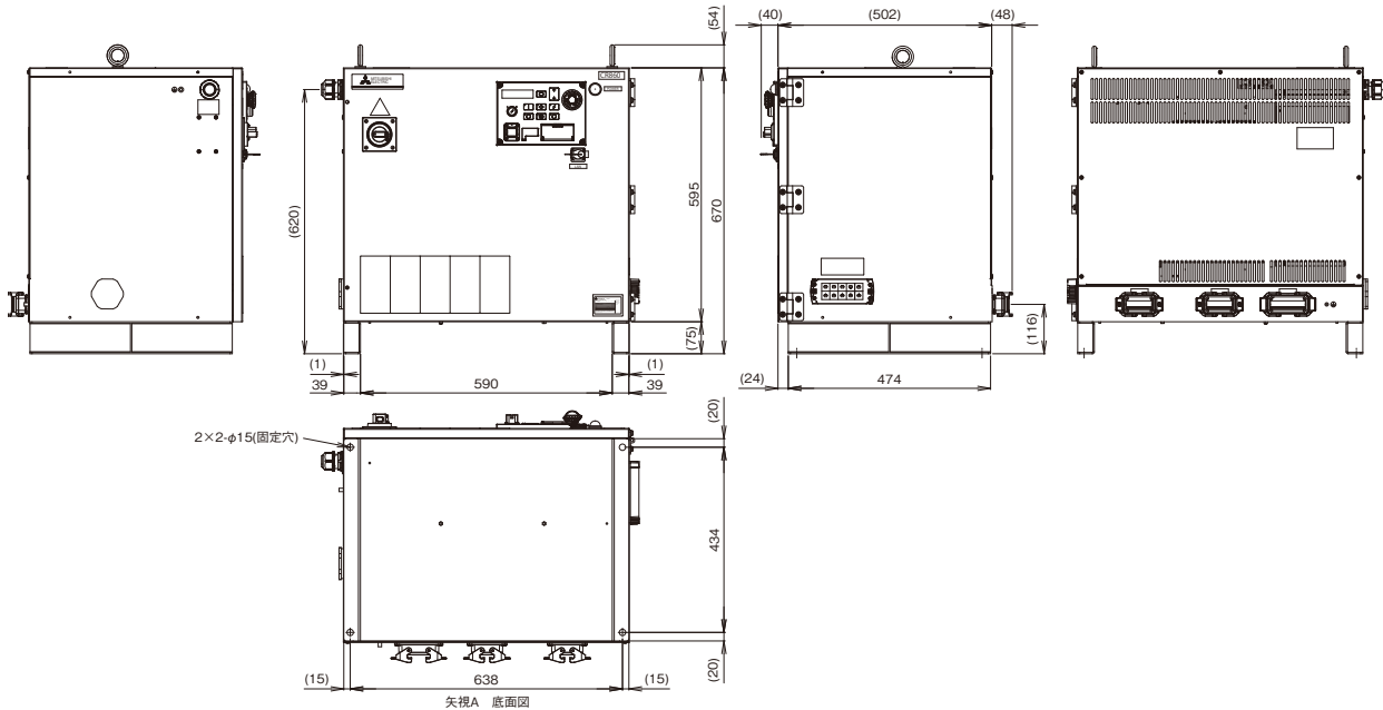
▶ 外形寸法図
