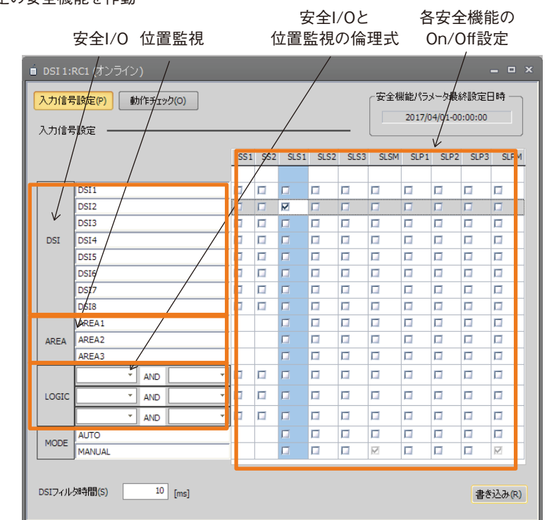
安全ロジック編集画面
