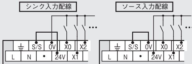
[AC電源タイプの入力配線図]
