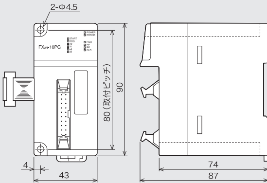
FX2N-10PG 質量: 約 0.2kg
