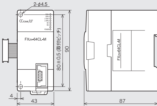
FX2N-64CL-M 質量: 約 0.15kg
