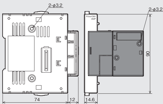
FX3G-CNV-ADP 質量：約 0.1kg
