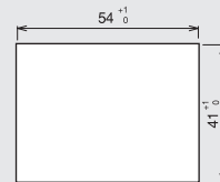
パネルカット寸法
