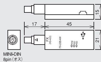
FX-USB-AW 質量：約 0.02kg (ケーブルを除く) 外装色：ブラウンスモーク
