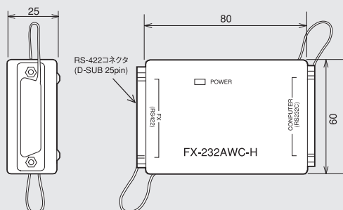
FX-232AWC-H 質量：約 0.1kg
