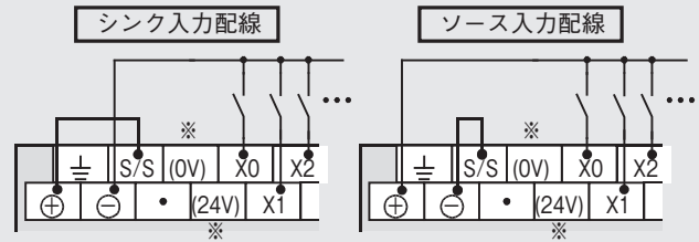
[DC電源タイプの入力配線図]
