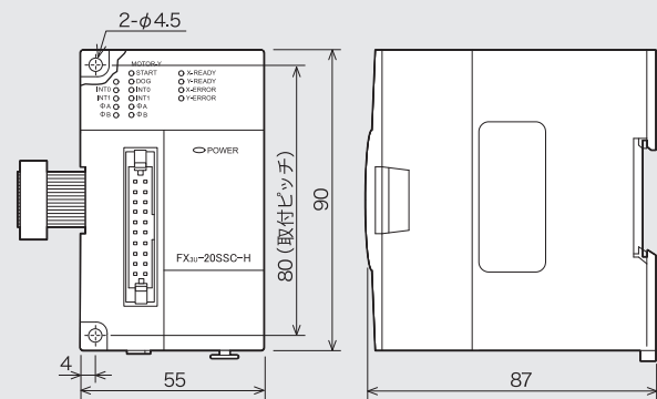
FX3U-20SSC-H 質量: 約 0.3kg
