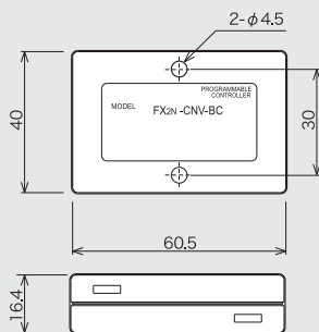
FX2N-CNV-BC 質量：約 0.04kg
