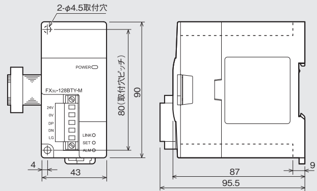
FX3U-128ASL-M 質量: 約 0.2kg FX3U-128BTY-M
