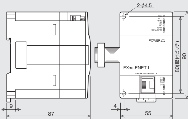
FX3U-ENET-L 質量: 約 0.3kg
