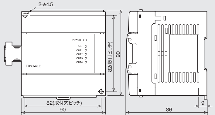
FX3U-4LC 質量: 約 0.4kg
