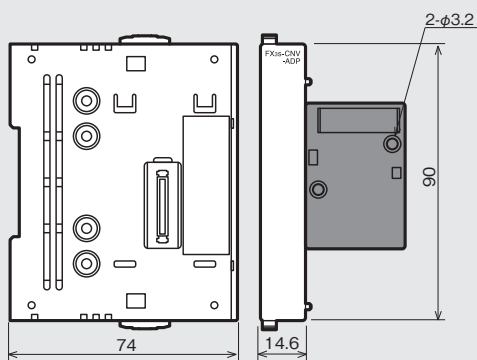
FX3s-CNV-ADP 質量：約 0.1kg
