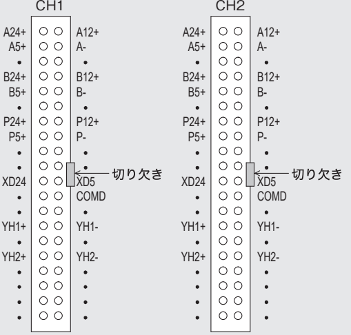
FX3U-2HC
