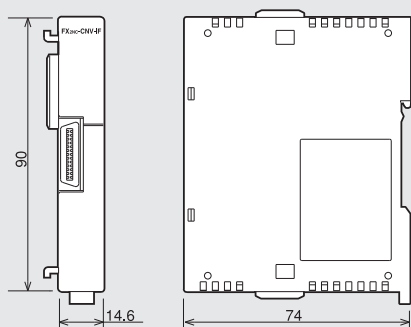
FX2NC-CNV-IF 質量：約 0.06kg
