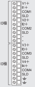
FX3UC-4AD
